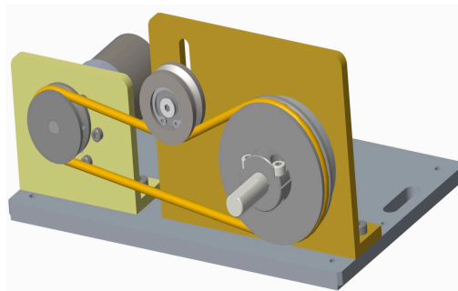
図1: 製品組立に用いるモデル製品(ベルトドライブユニット)
